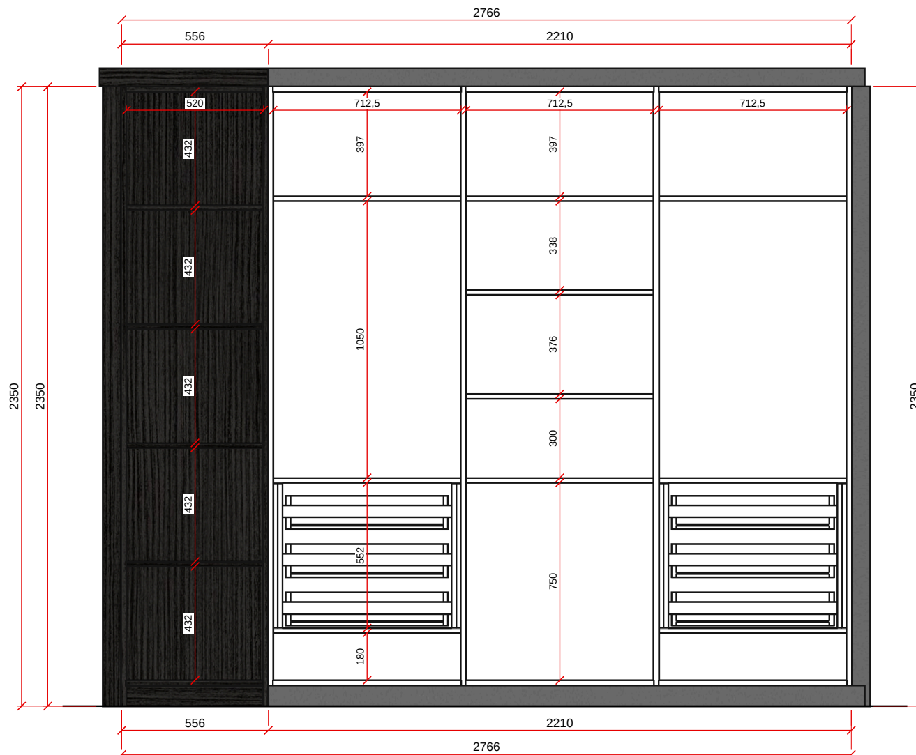
VISTA A - ESC. 1:20
